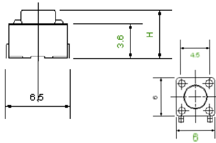
TMR114A
